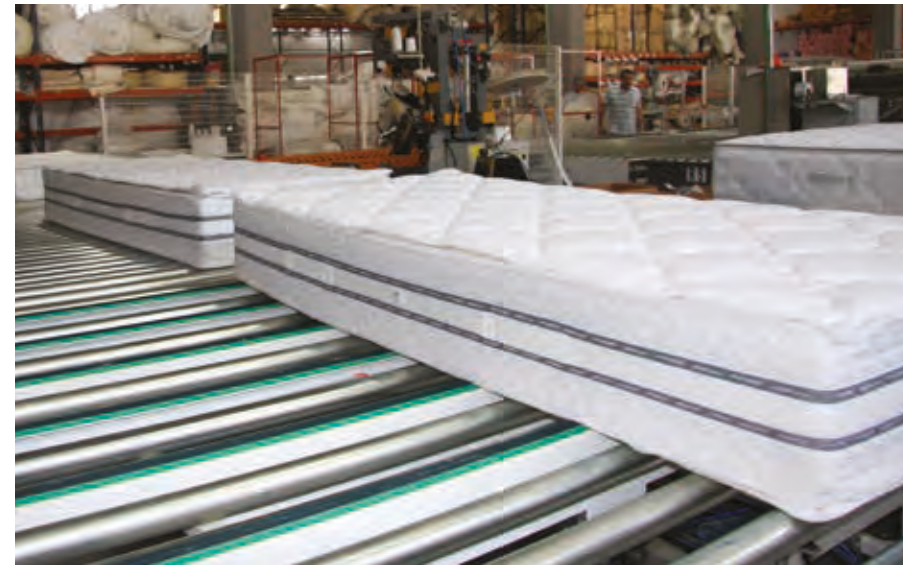
Μεταφορά των στρώματων στις μηχανές ρελιάσματος. The mattresses are transferred to the hemming machines.
